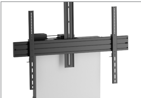
VESA, min. 300 x 200 mm - max. 900 x 600 mm
